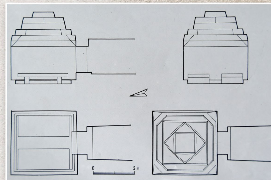
Plan géométral de la chambre funéraire.
