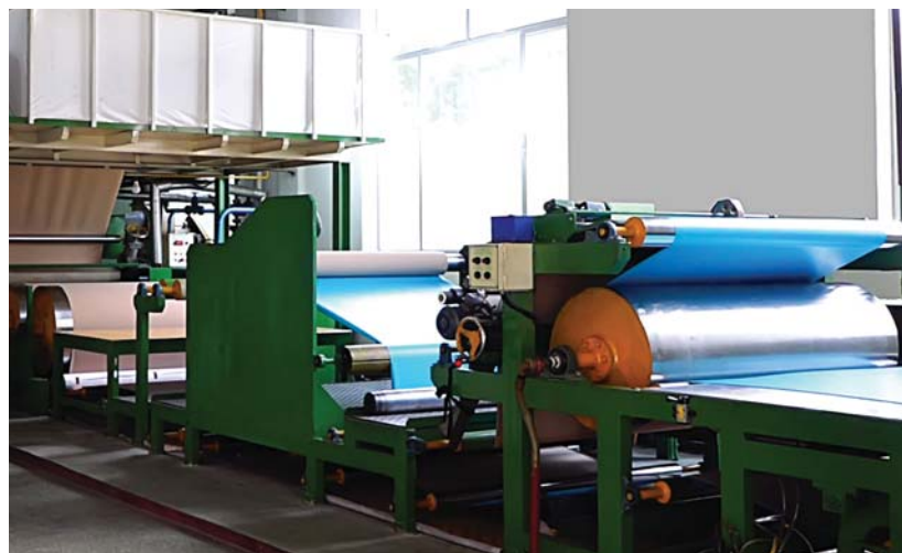
Процесс производства синтетических кож методом сухого покрытия.
